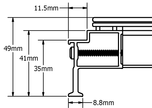
Figure 4: Long Edge Frame Detail
